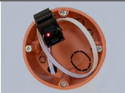
PLUG-ON OL-SMI KEYSTONE MODULE
